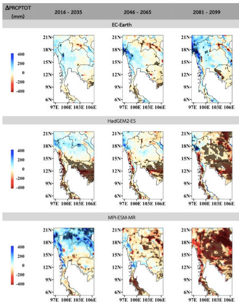
รูปที่ 1-8 การคาดการณ์ปริมาณฝนรวมรายปี (PRCPTOT) ภายใต้ภาพสถานการณ์จำลอง RCP 4.5
